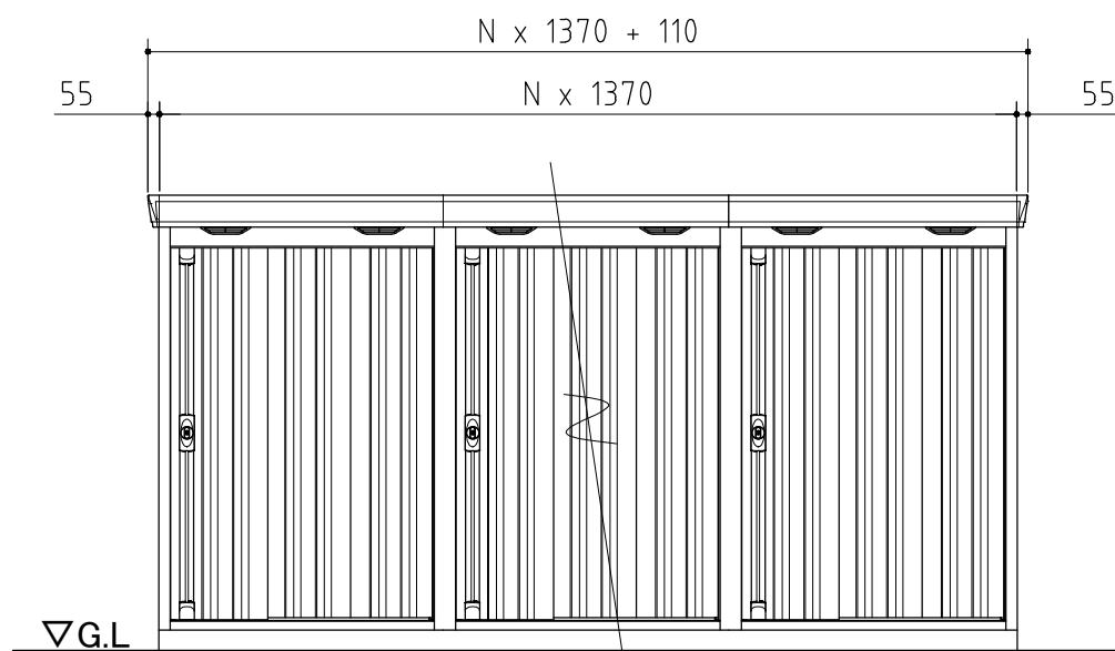
正面図
